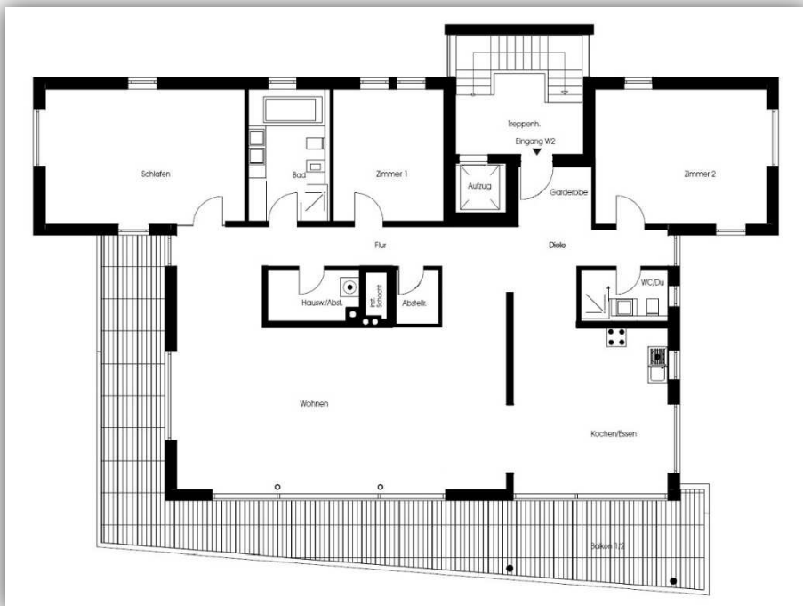
12: GRUNDRISS
